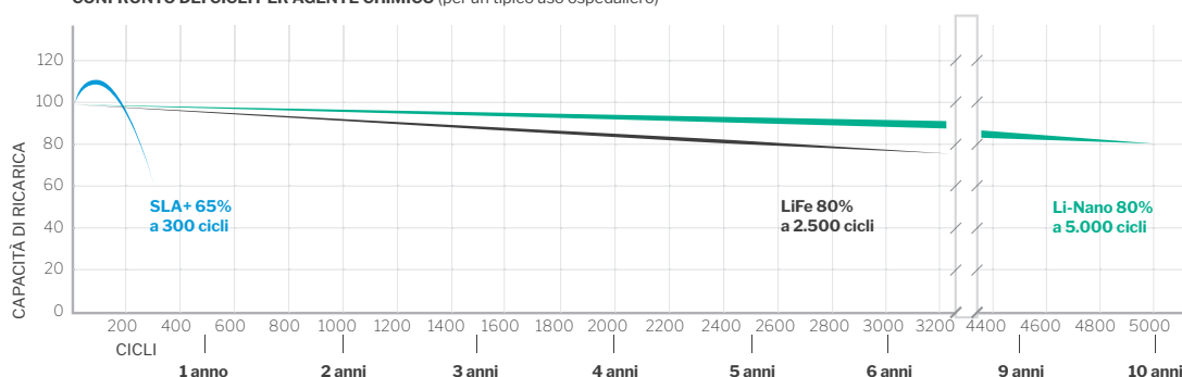
CONFRONTO DEI CICLI PER AGENTE CHIMICO (per un tipico uso ospedaliero)
